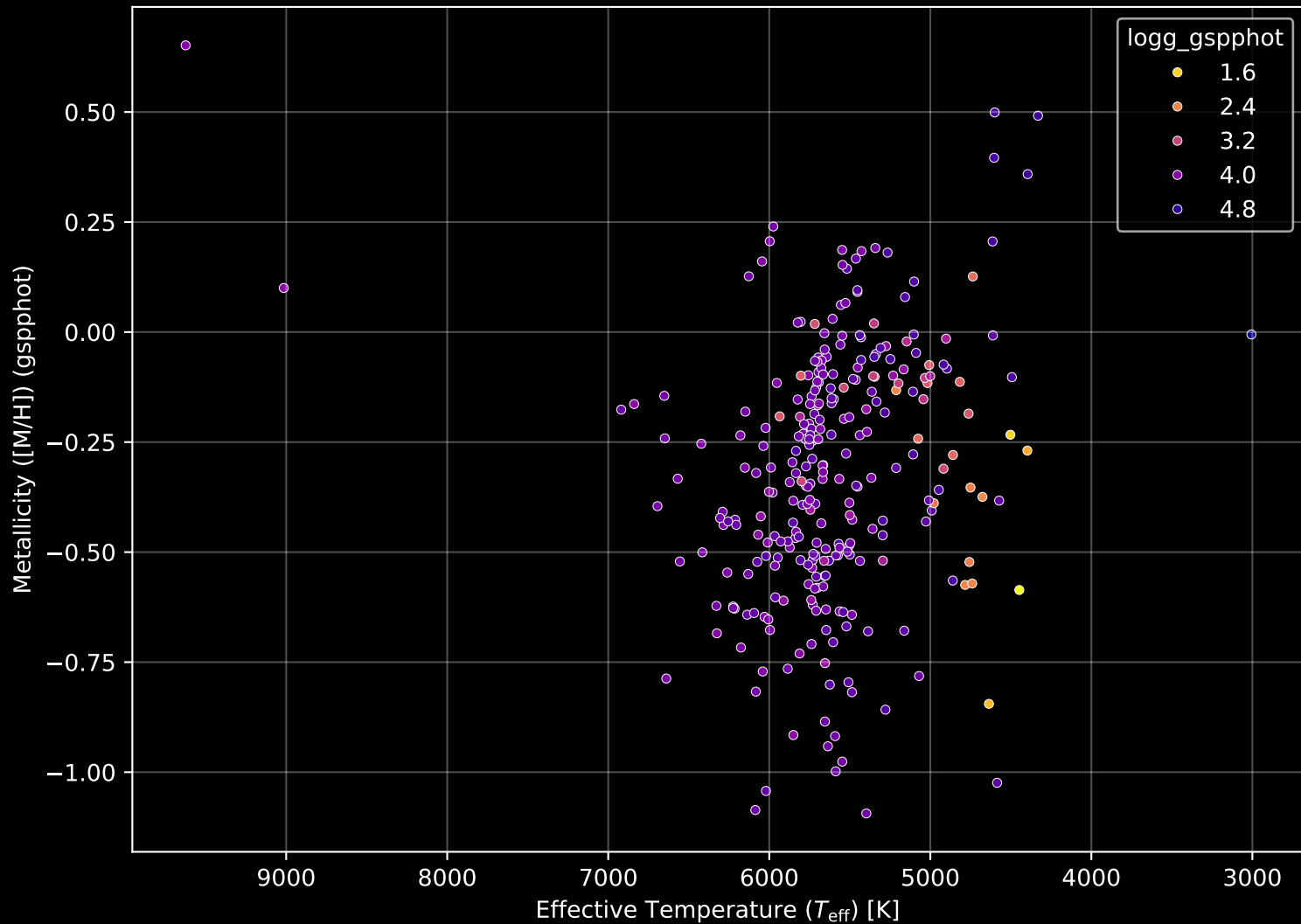
GALAH DR4 Field: [202] Stellar Population Parameters (n= 288)
