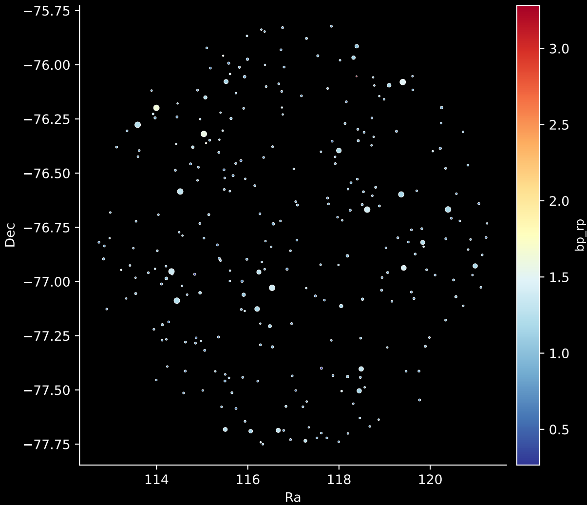
GALAH DR4 Field: [202] Stars: 288
