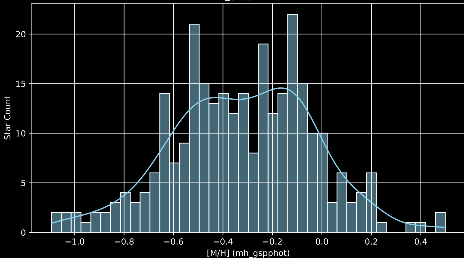
GALAH DR4 Field: [202] [M/H] (mh_gspphot) (n= 287)
